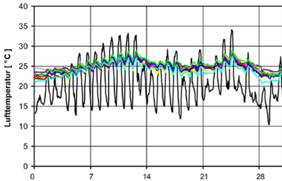
Tagesgang der Außenlufttemperatur (schwarz) und der mittleren Gebäudetemperaturen der 9 Niedrigenergiehäuser (farbig) im August nach [1].
