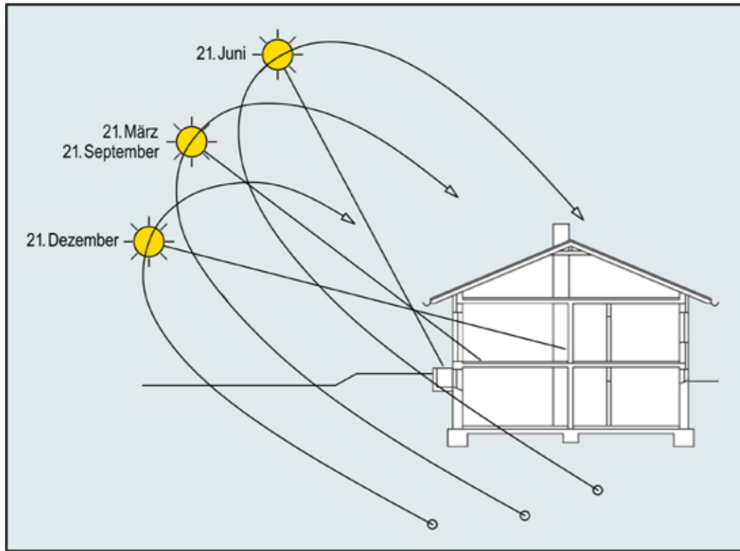
Sonnenhöchststände im Jahresverlauf.
