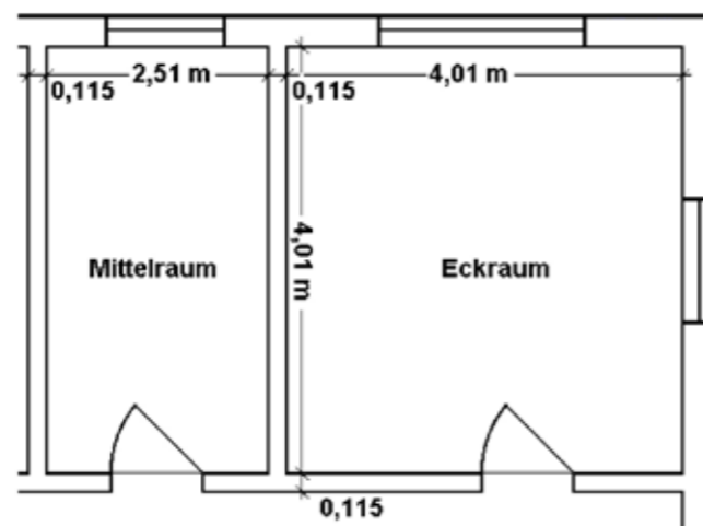
Den Musterrechnungen zugrunde liegende Raumanordnung
