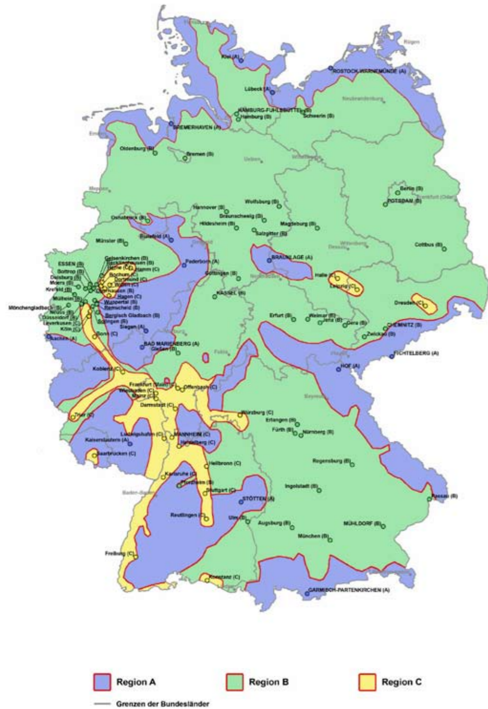
Sommerklimaregionen nach DIN 4108-2
